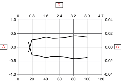
Fig. 4 Fast mode
